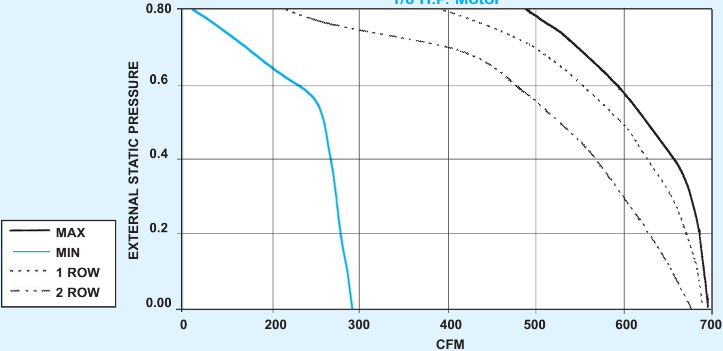
FAN SIZE C - UNDERFLOOR AC U3 1/6 H.P. Motor
